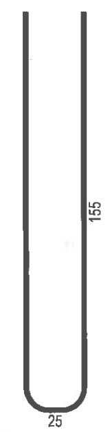
5 4ø12 L=3.35m
