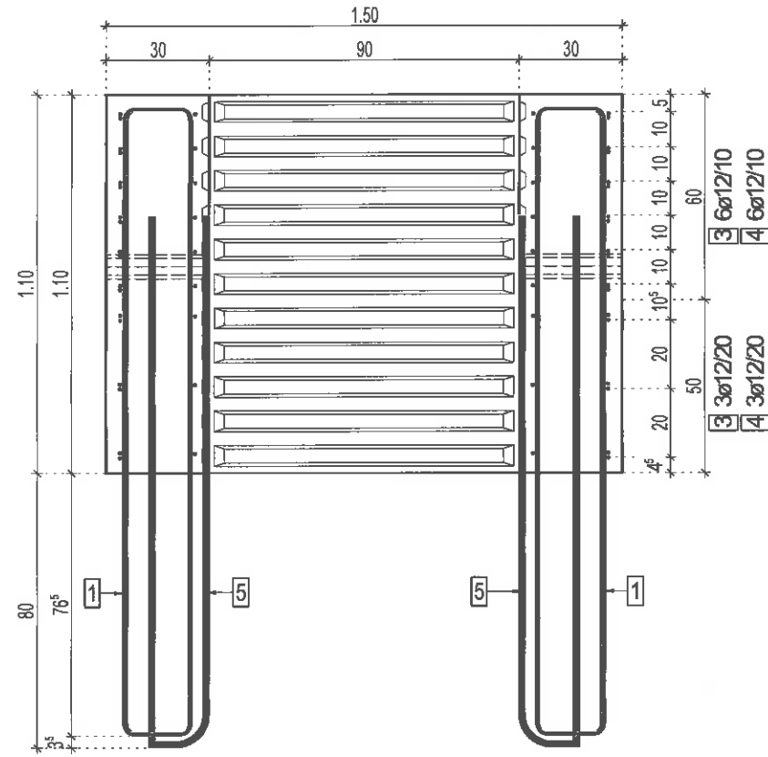
SECTIUNEA A-A
