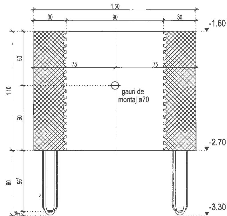
SECTIUNEA B-B
