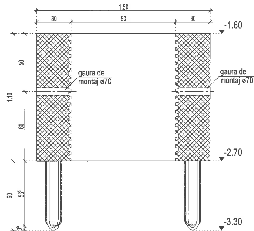
SECTIUNEA A-A
