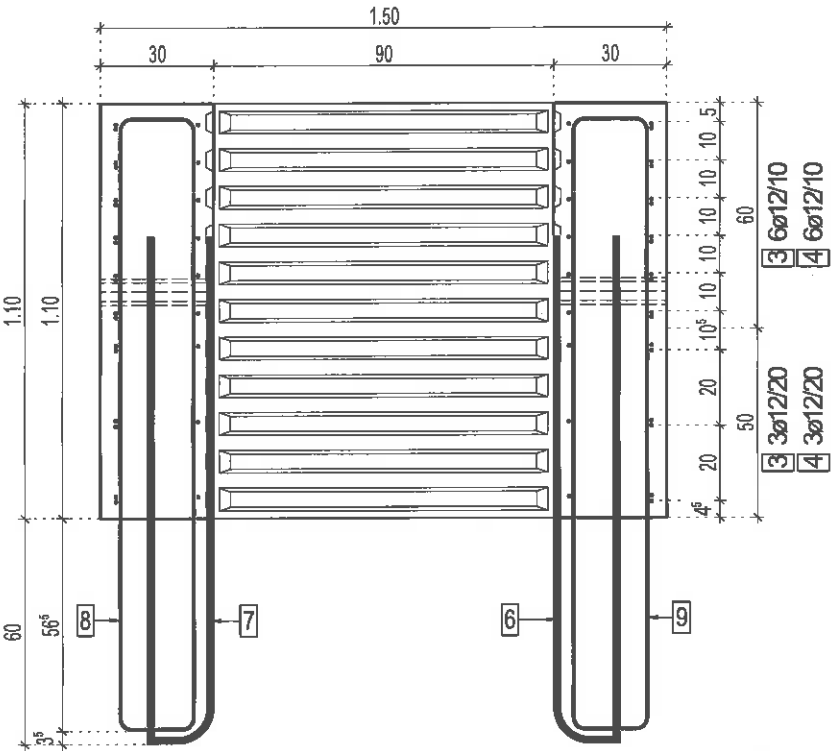
SECTIUNEA A-A
